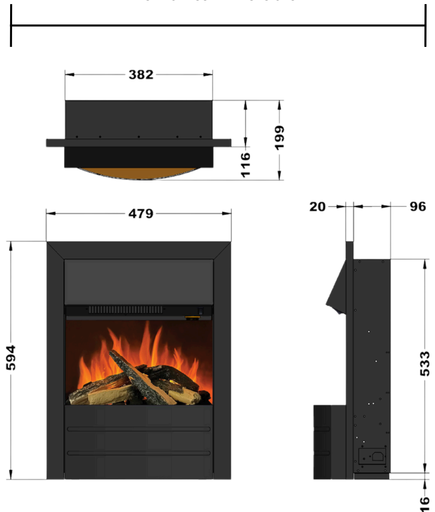
ilektro Insert Dimensions
